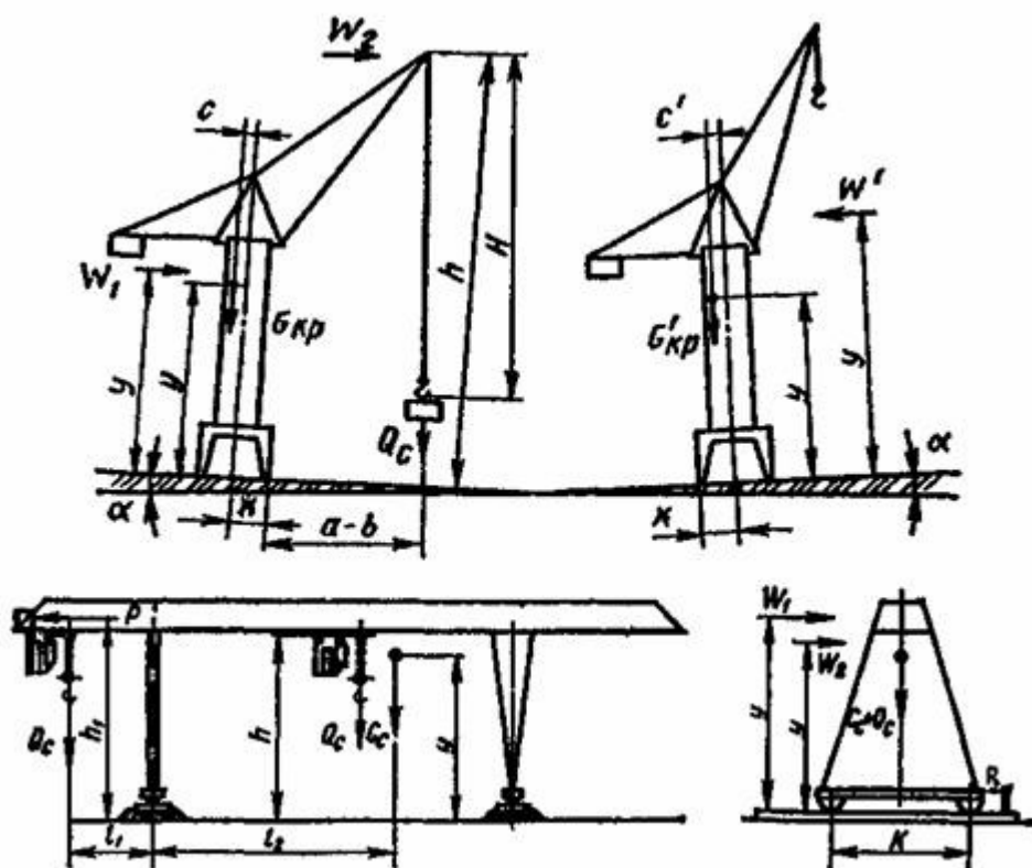
Рис. 1. Схема расположения нагрузок действующих на кран.
