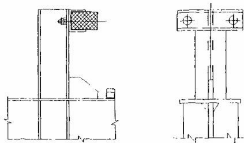
Рис. П.9.5. Общий вид тупикового упора ударного типа устанавливаемого на металлических балках.
