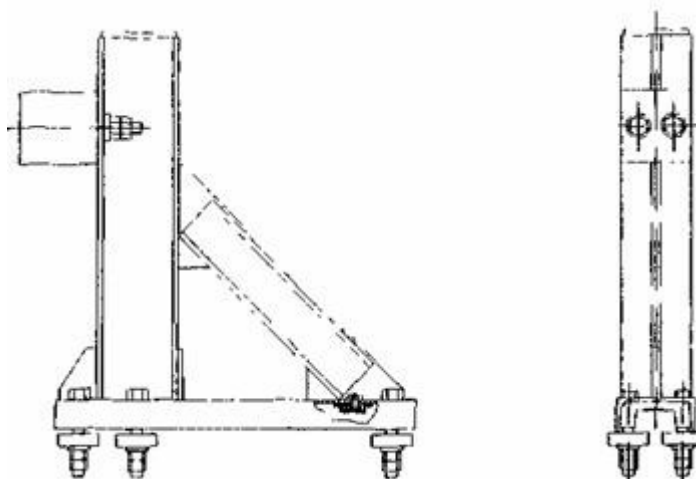
Рис. П.9.4. Общий вид тупикового упора ударного типа (разработчик НПЦ «Путь К», шифр 030-02.00.000)
