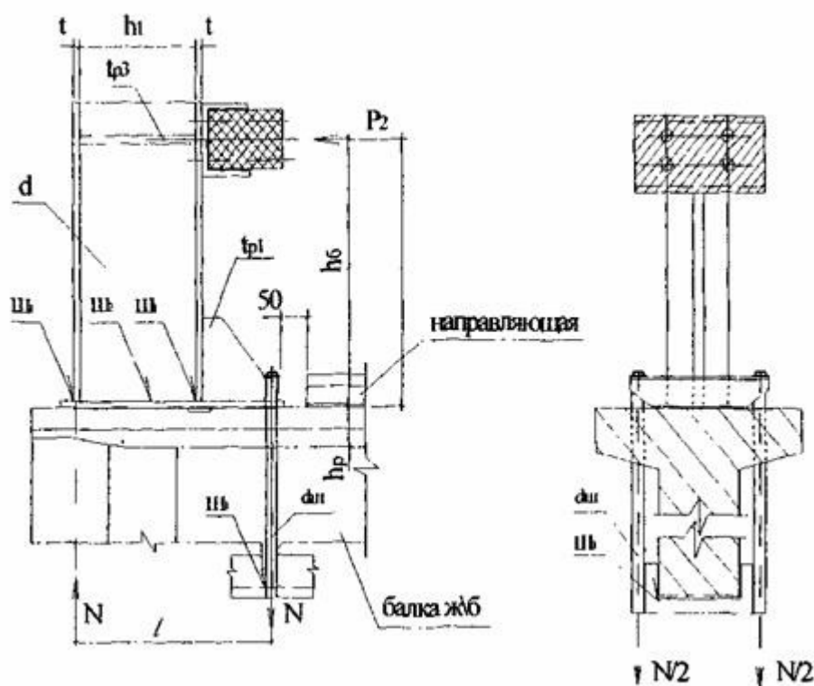
Рис. 3. Расчетная схема тупикового упора на железобетонной балке:
