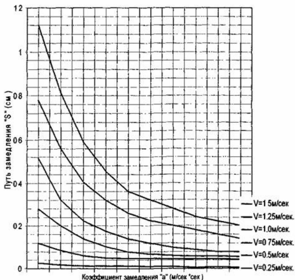
Рис. 5. Зависимость коэффициента и пути замедления от скорости движения крана
