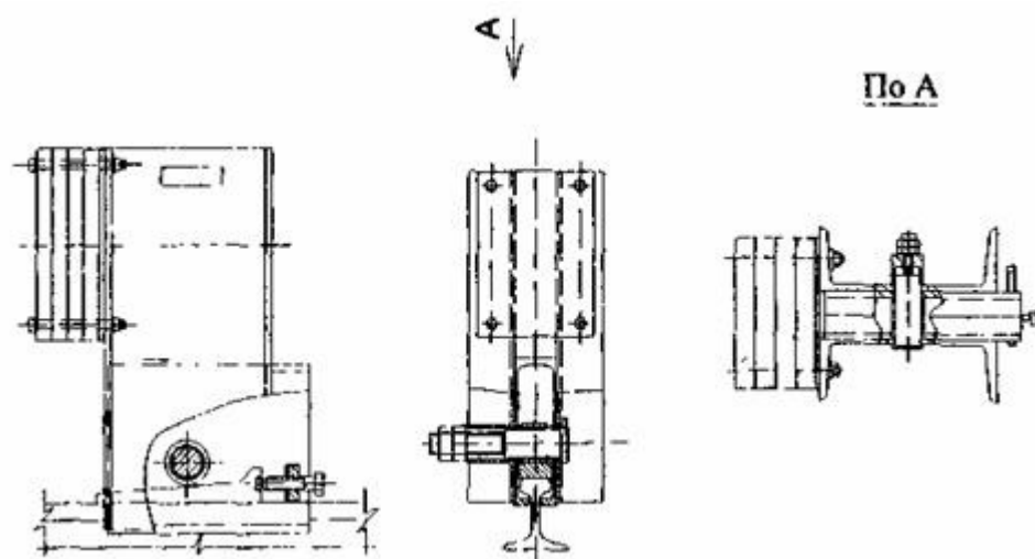
Рис. П.9.3. Общий вид тупикового упора ударного типа (разработчик Механический завод УКР, шифр проекта - КБ-503А.23.04.00)
