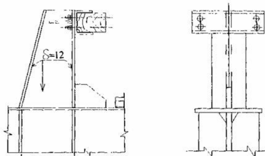
Рис. П.9.6. Общий вид тупикового упора ударного типа устанавливаемого на металлических балках.
