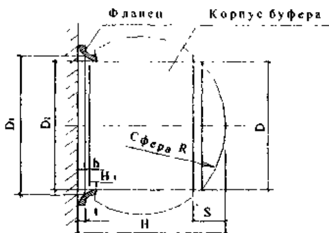
Рис. 4. Общий вид с обозначением параметров резиновых буферов
