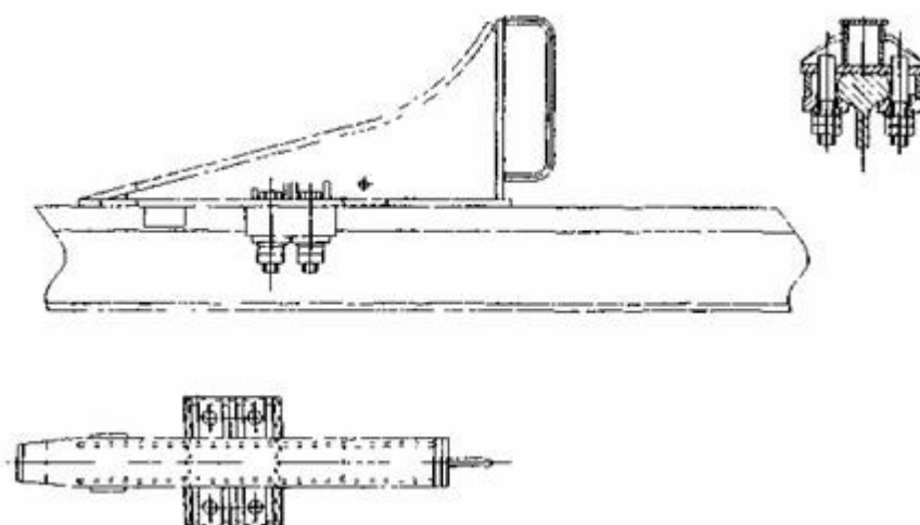
Рис. П.9.2. Общий вид тупикового упора безударного типа (разработчик НПЦ «Путь К», спецификация шифр проекта 030-01.00.00)
