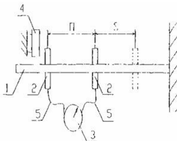
Рис. 6. Установка для определения скорости движения крана и расстояния проходимого краном до полной остановки от начала взаимодействия с упором.
