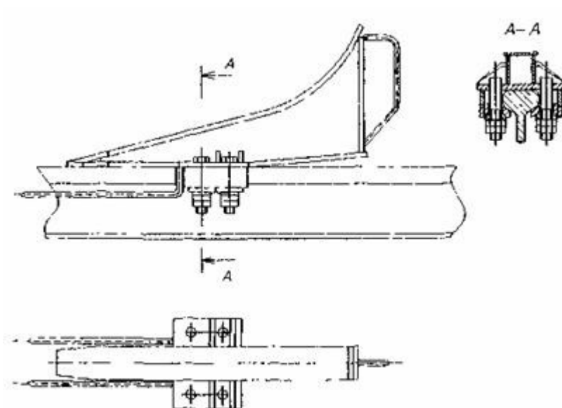
Рис. П.9.1. Общий вид тупикового упора безударного типа (разработчик ЦНИИОМТП, шифр проекта 29-4.00.000)
