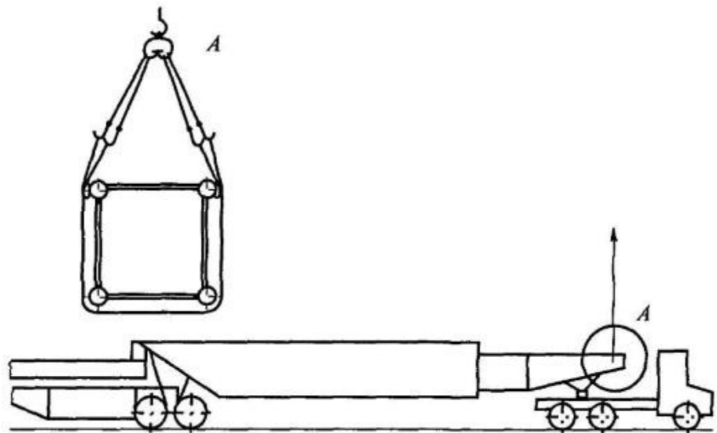
Схема 3. Стрповка башни крана за оголовок при снятии крана с тягача
