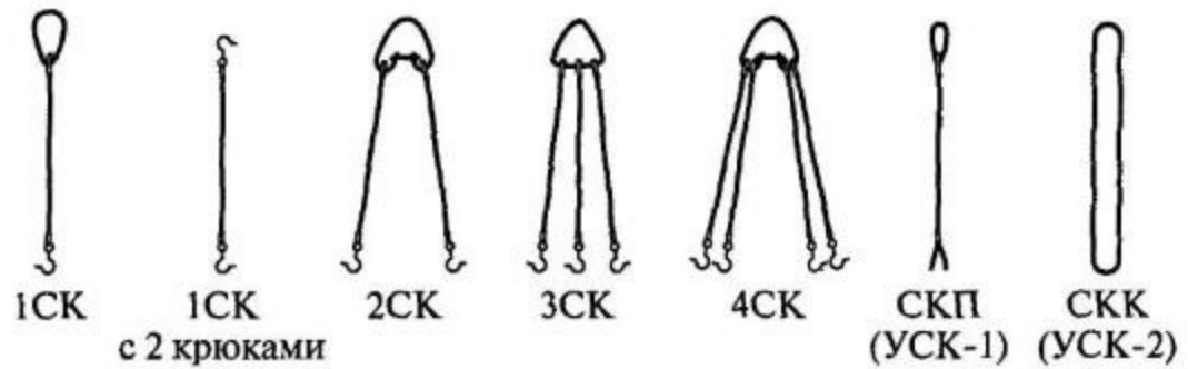
Рис. 32. Виды стропов:
