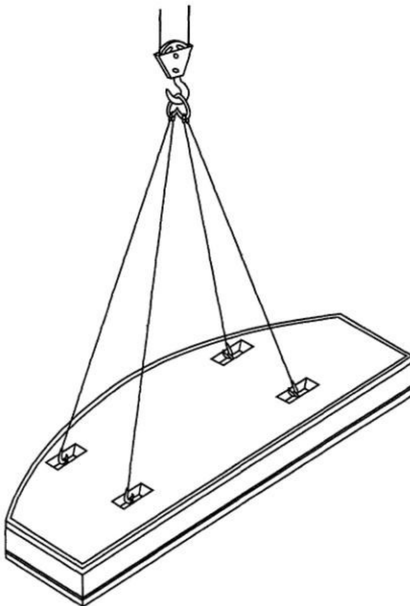
Схема 10. Строповка плиты противовеса
