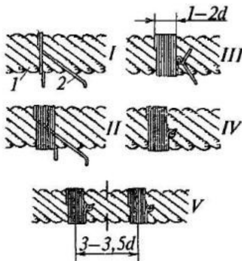
Рис. 30. Последовательность обвязки (I-V) каната перед рубкой: 1 - канат; 2 - проволока; 3 - место рубки
