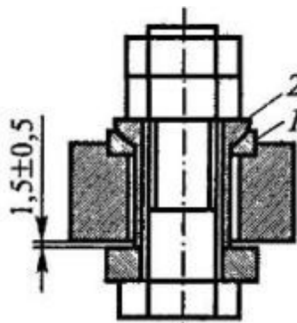
Рис. 13. Схема крепления лебедки при ее трехточечном опирании: 1 - сферическая втулка; 2 - шайба
