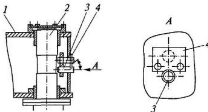
Рис. 15. Фиксация ходовых тележек во флюгере: 1 - флюгер; 2 - шкворень ходовой тележки; 3 - переставной палец (верхнее положение - при перевозке, нижнее положение - для работы); 4 - оседержатель
