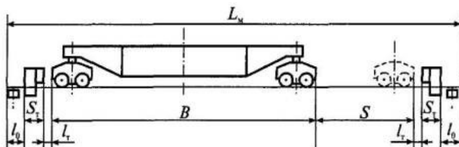
Рис. 6. К расчету длины монтажного участка пути
