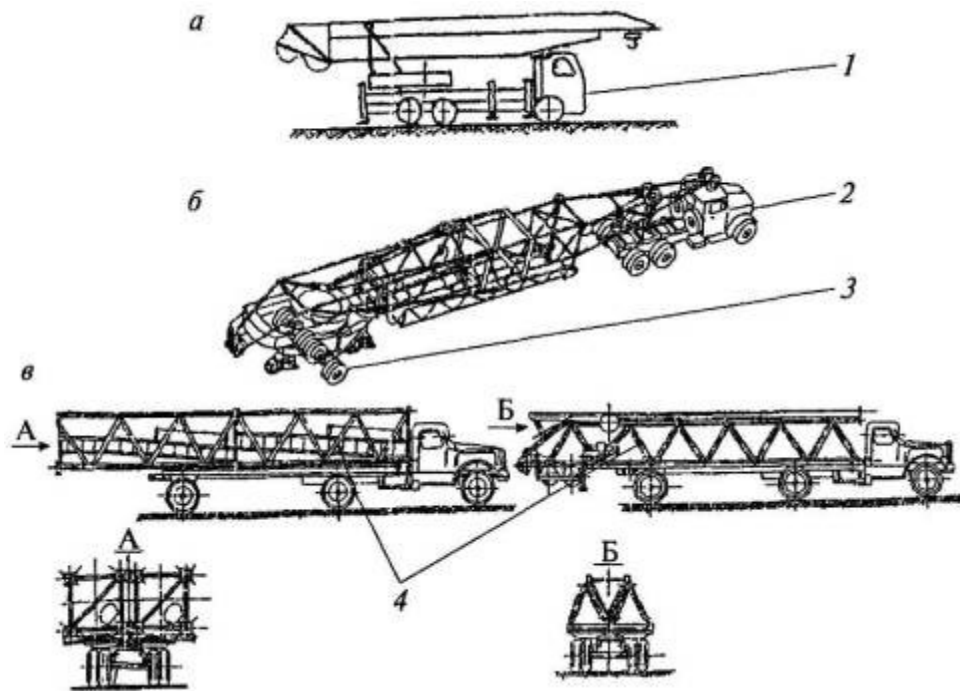
Рис. 1. Схемы перевозки и завоза (заезда) кранов к месту монтажа: а - быстромонтируемого крана; б - крана в мобильном исполнении; в - крана с разборкой на узлы;
