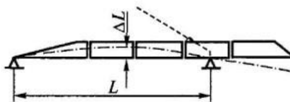
Рис. 20. Схема к определению прямолинейности собранной из секций стрелы
