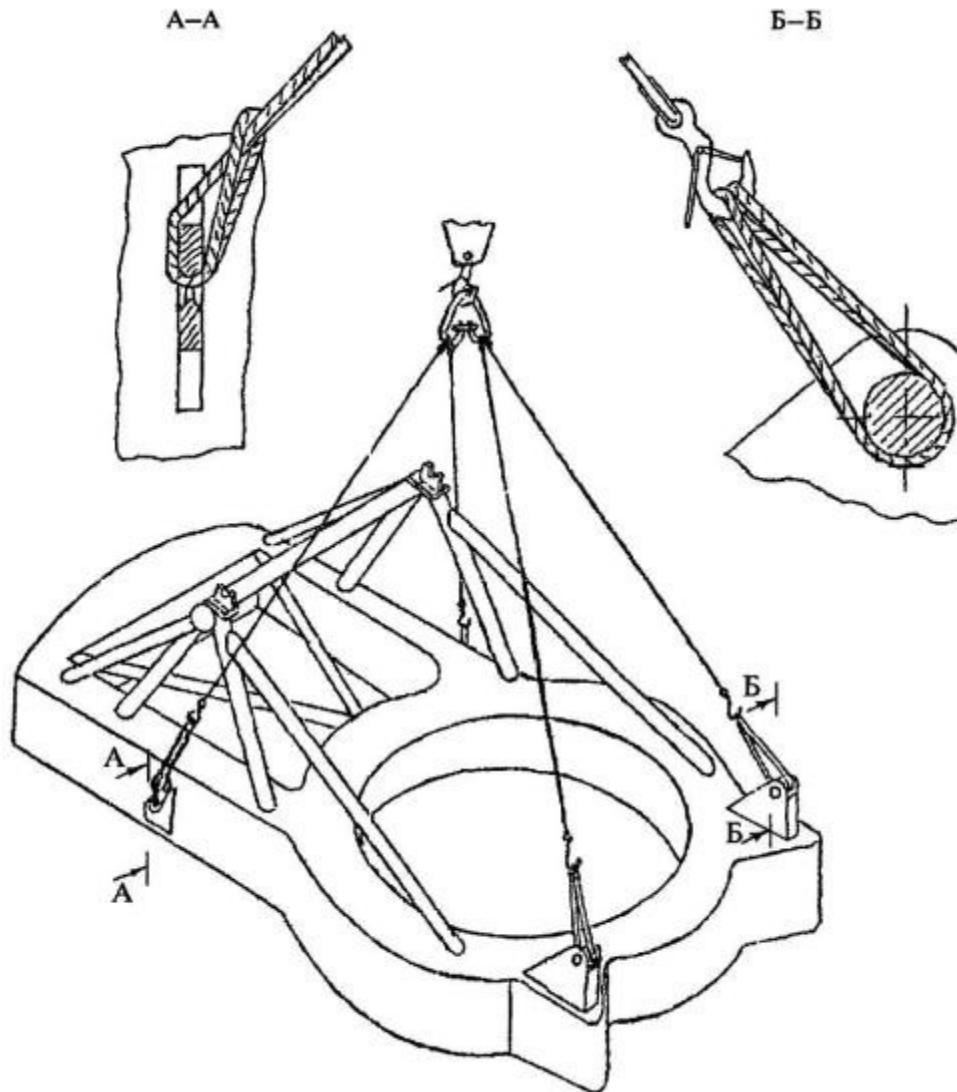
Схема 2. Строповка поворотной платформы
