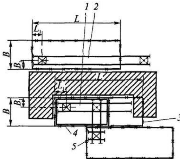
Рис. 8. К выбору башенного крана:
