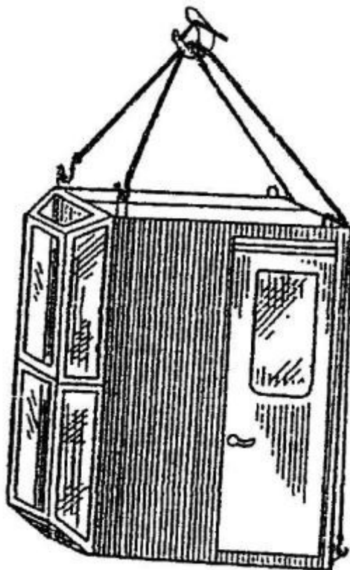
Схема 11. Строповка кабины (в случае необходимости ее кантования)
