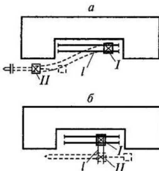
Рис. 34. Способы вывода крана из стесненных условий: а - с переводом на пересекающийся путь; б - с передвижкой пути; I, II - положения крана на путях; I - рельсовый путь
