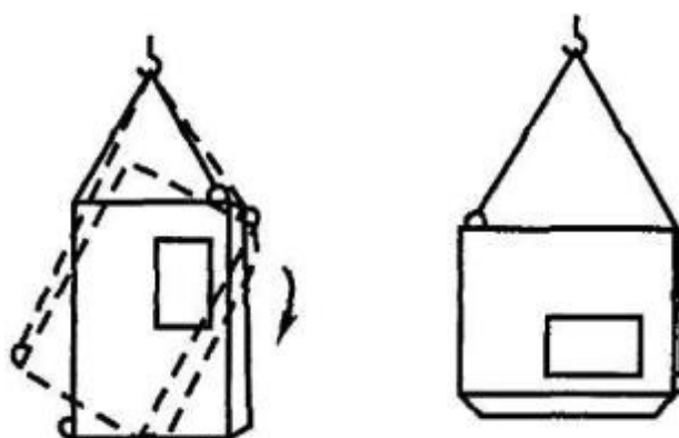
Рис. 17. Схема кантования кабины
