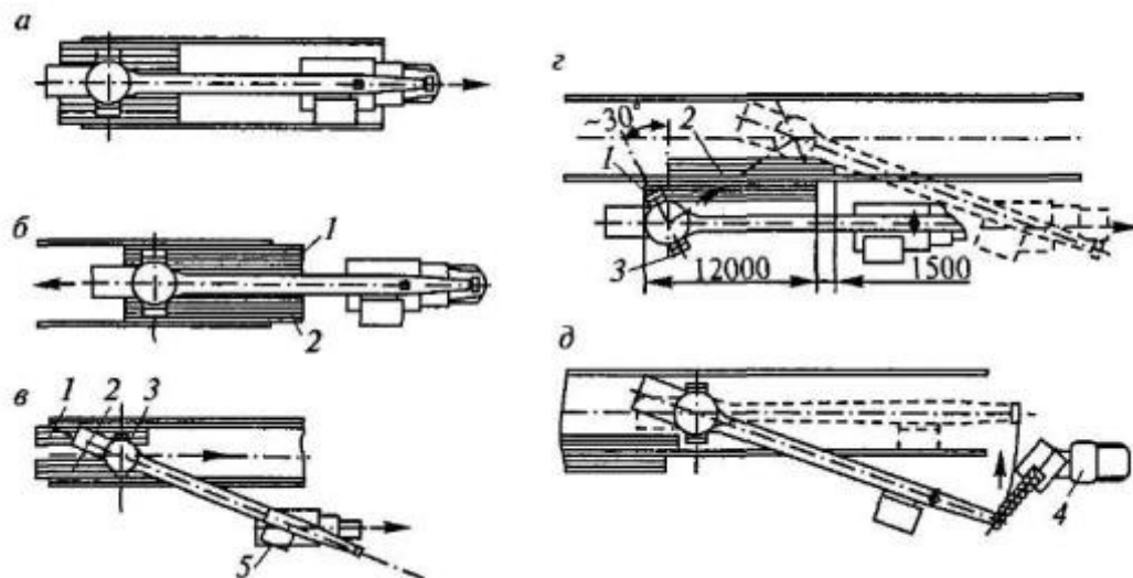
Рис. 12. Способы завоза на рельсовый путь крана в мобильном исполнении: а - при движении тягача по пути вперед; б - при движении тягача задним ходом; в - при движении тягача сбоку пути, с заездом основания крана с торца пути; г - то же, с переездом основания крана через пути; д - перемещение башни крана в монтажное положение по оси пути; 1, 2 - щиты; 3 - подкатная тележка; 4 - стреловой кран; 5 - тягач
