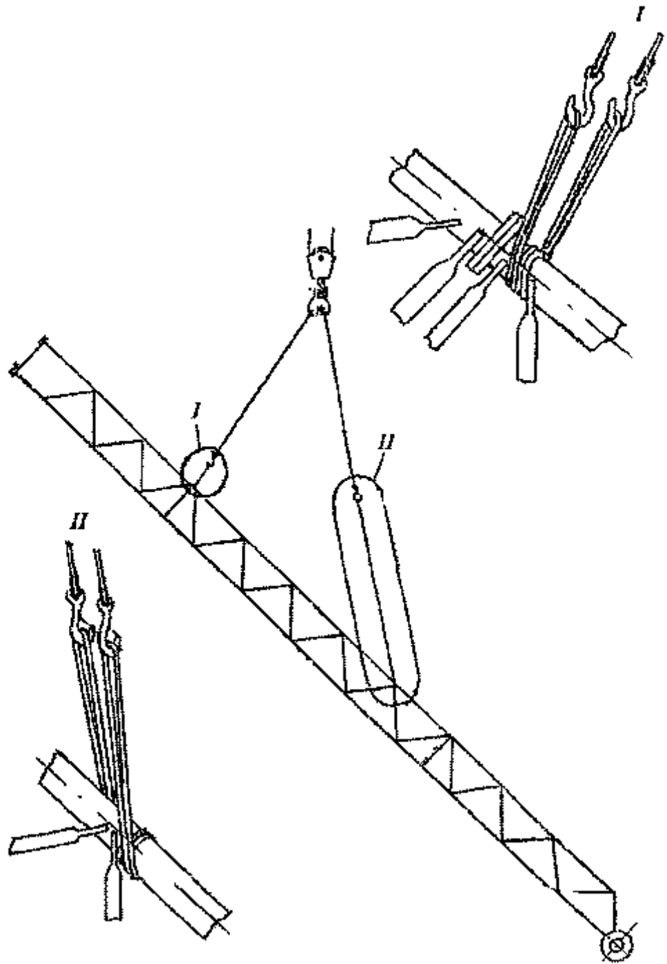
Схема 6. Строповка стрелы в сборе при навешивании на башню
