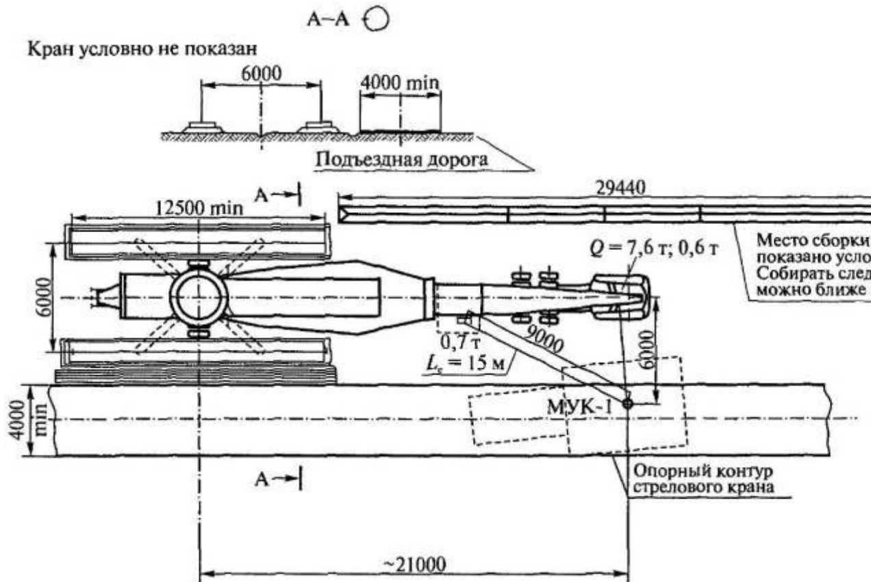
Рис. 3. Схема мест установки крана КС-45717 при монтаже после мобильной перевозки крана типа КБ-403:
