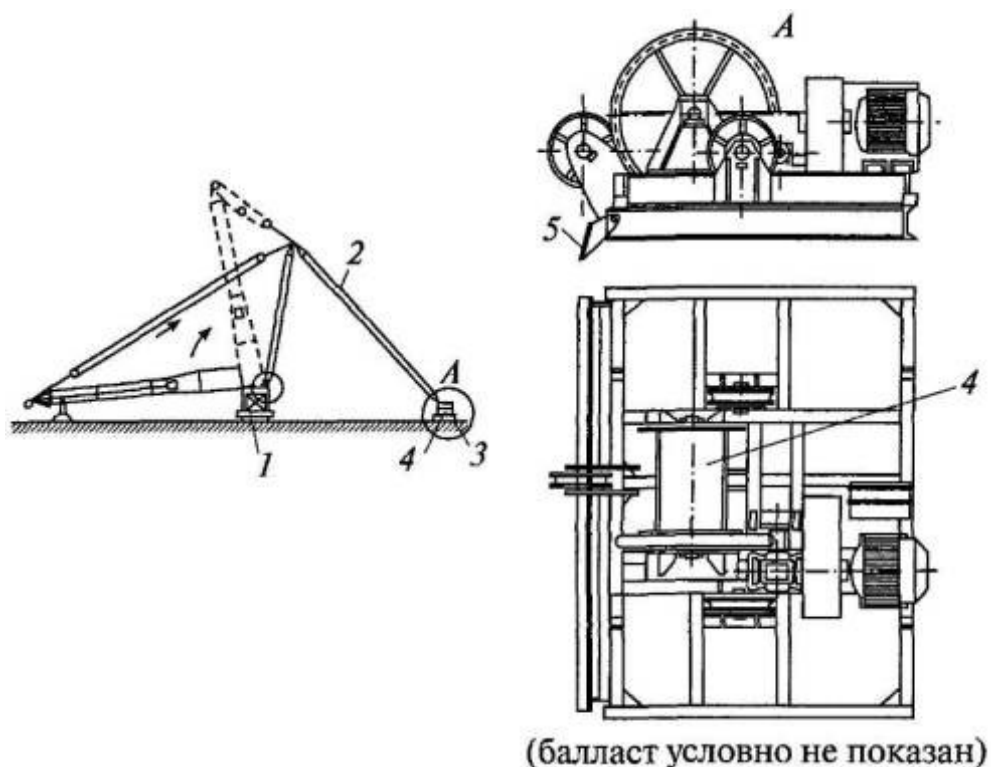
Рис. 10. Установка якорных устройств:
