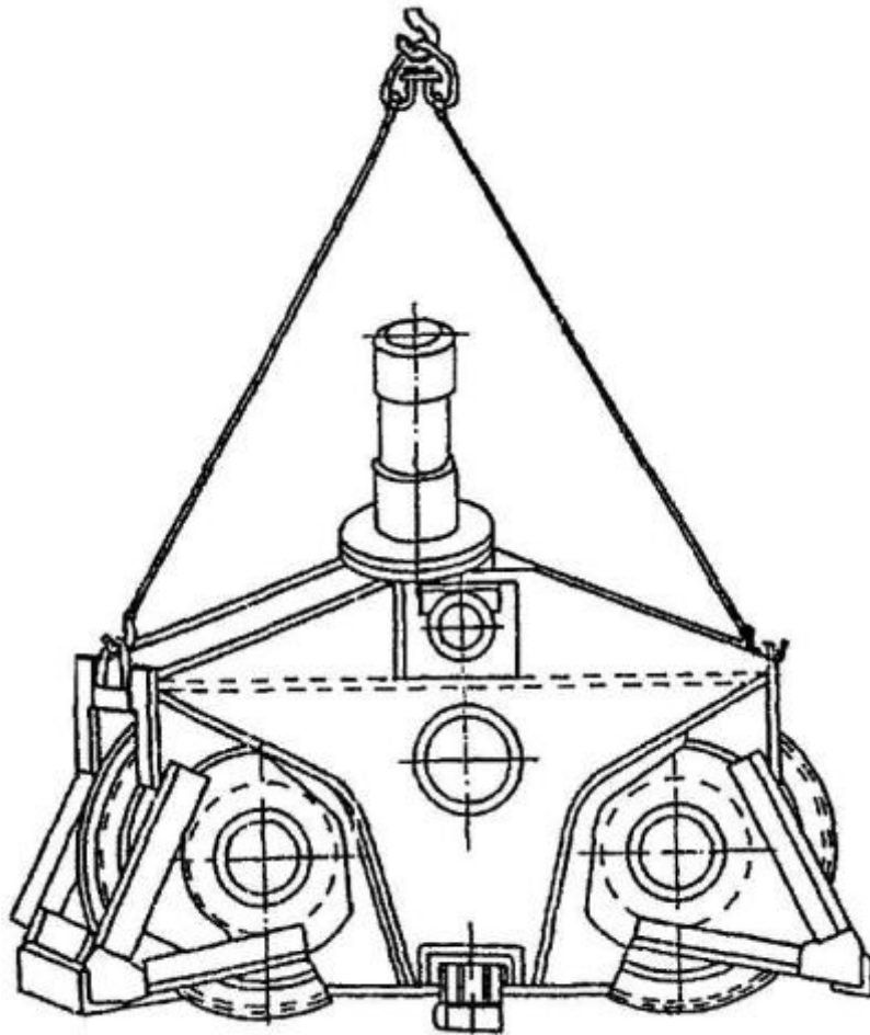
Схема 8. Строповка ходовой тележки
