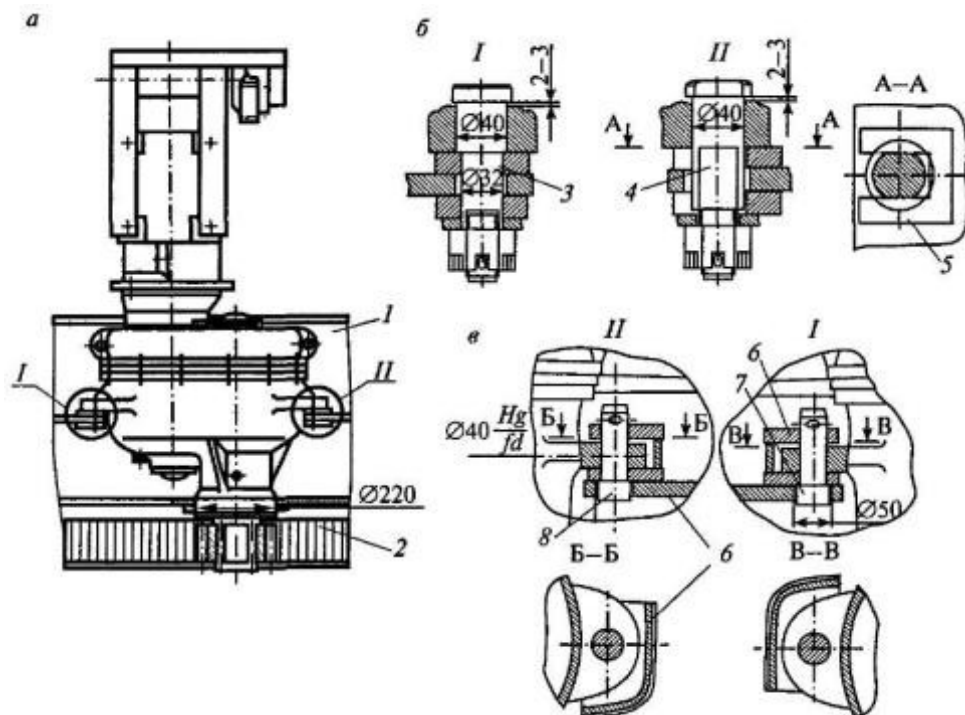
Рис. 14. Схема крепления механизма поворота: а - общий вид механизма; б - для кранов, не имеющих вильчатых кронштейнов; в - для кранов с вильчатыми кронштейнами; 7 - поворотная платформа; 2 - ОПУ; 3 - 4 - специальные пальцы; 5 - шайба; 6 - вильчатый кронштейн; 7 - 8 – пальцы
