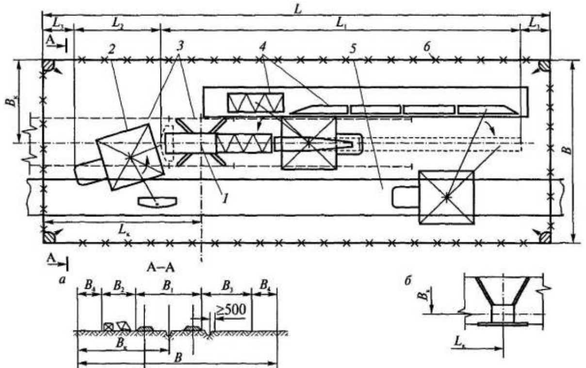
Рис. 2. К определению размеров монтажной площадки на период монтажа: а - при симметричном расположении башни относительно рельсового пути; б - при асимметричном расположении;
