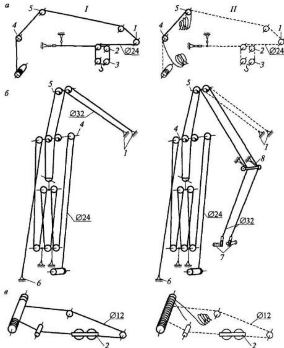
Рис. 26. Схема запасовки канатов (на примере крана КБ-403):
