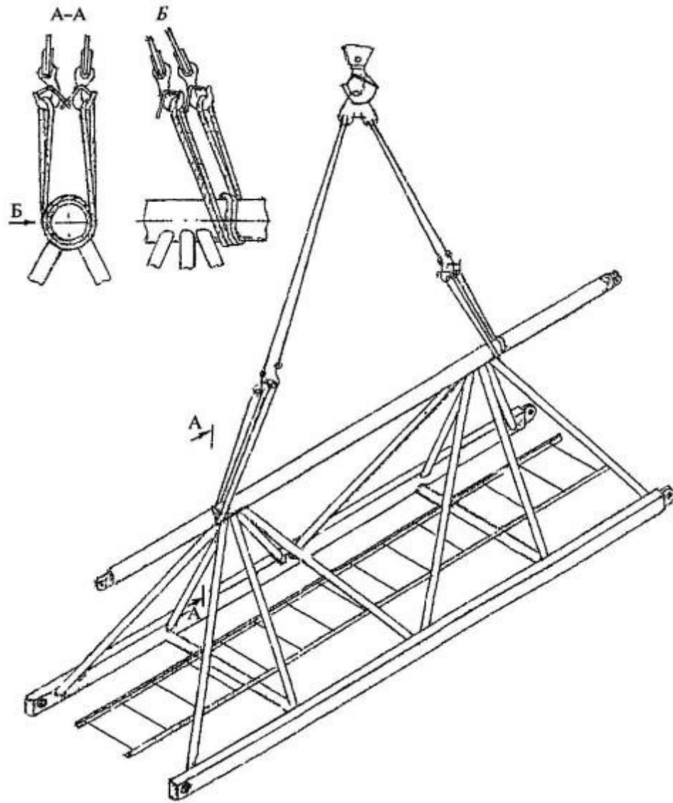
Схема 5. Строповка секции стрелы
