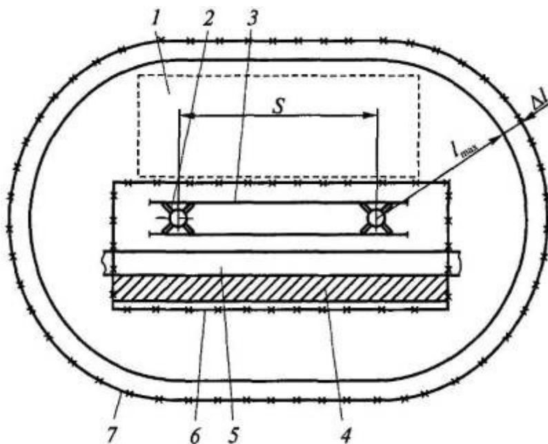
Рис. 4. Определение опасной зоны на период испытания крана: 1 - место возводимого здания; 2 - кран; 3 - рельсовый путь; 4 - место для складирования элементов; 5 - дорога для автотранспорта; 6 - монтажная площадка; S - возможная зона передвижения крана
