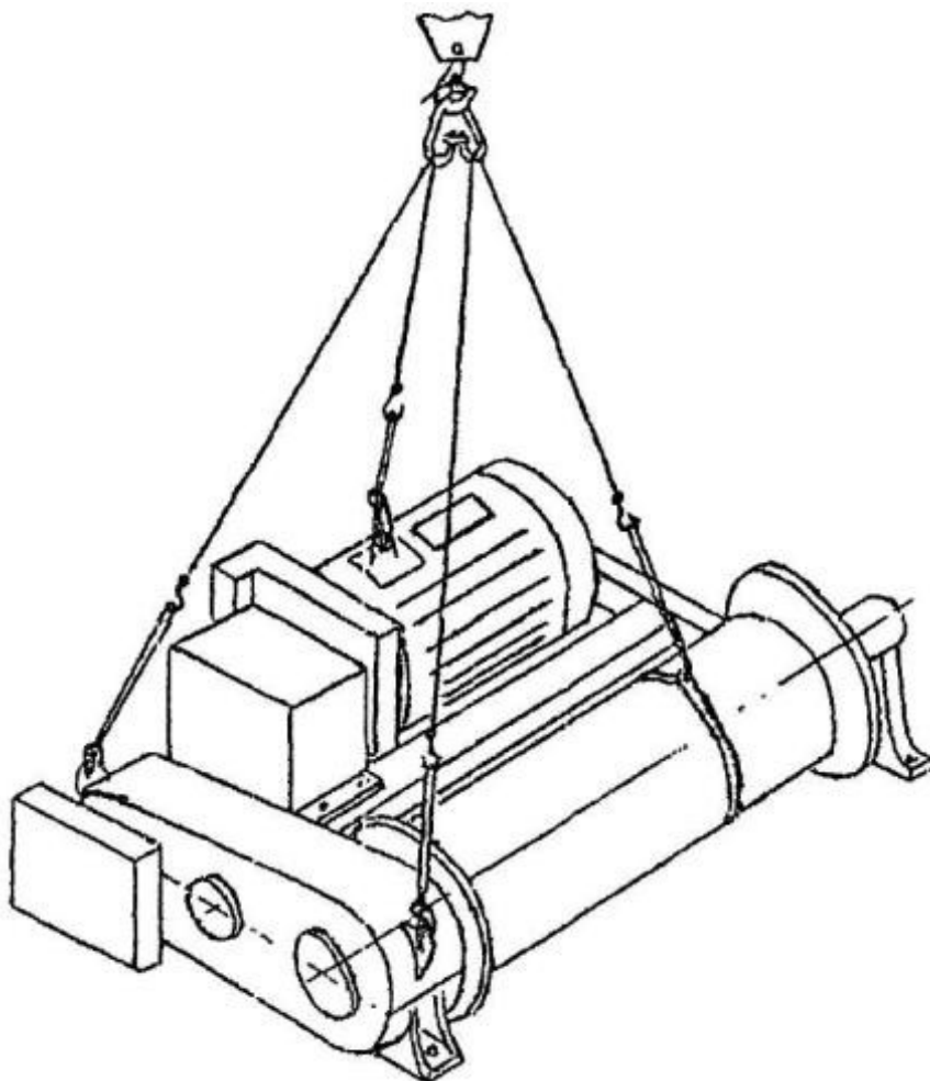
Схема 7. Строповка грузовой лебедки
