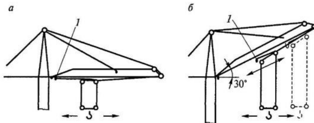
Рис. 25. Схема запасовки грузового каната: а - при работе с горизонтальной стрелой; б - то же, со стрелой под уклоном 30^\circ ; 1 - точка крепления грузового каната
