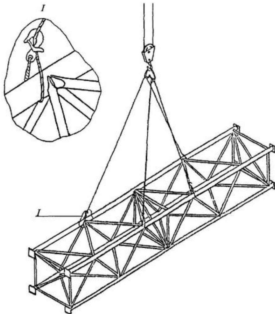
Схема 4. Стрповка секции башни
