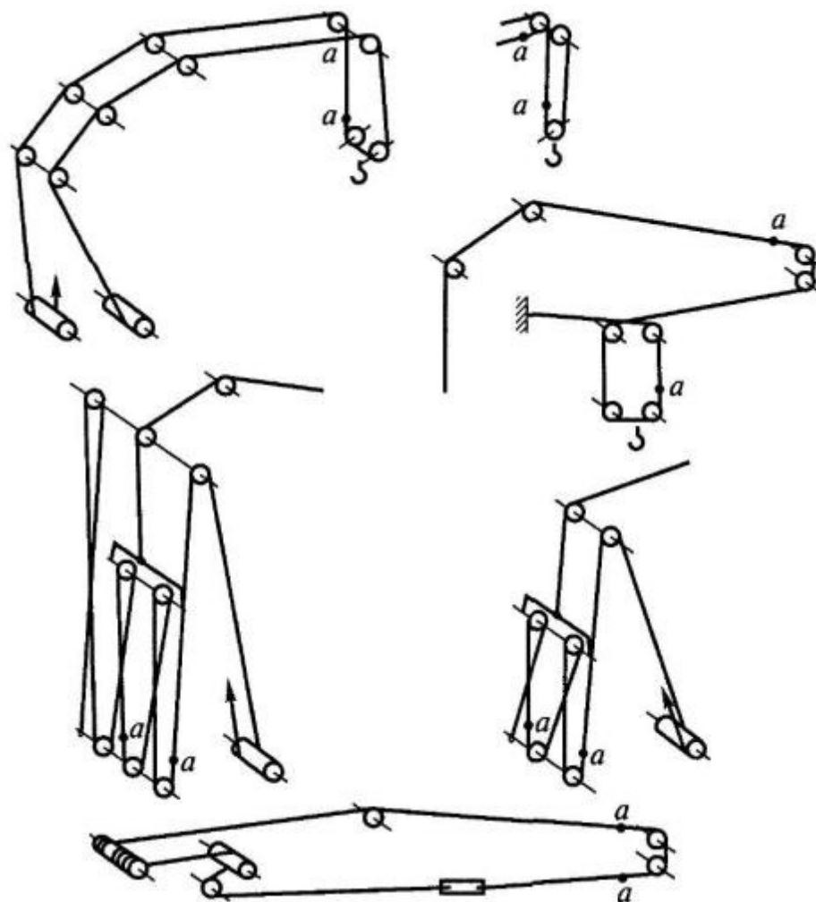
Рис. 29. Типовые схемы запасовки канатов:
