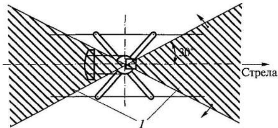
Рис. 35. Расположение подвижной зоны 1 непосредственной опасности
