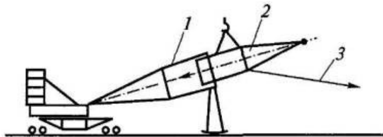
Рис. 5. Монтаж верхней секции с оголовком: 1 - портал башни; 2 - верхняя секция с оголовком; 3 - оттяжка
