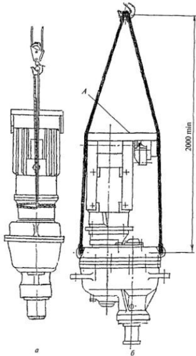
Схема 9. Строповка механизма поворота: а - с планетарным редуктором; б - с цилиндрическим редуктором; А - перед строповкой открыть кожух
