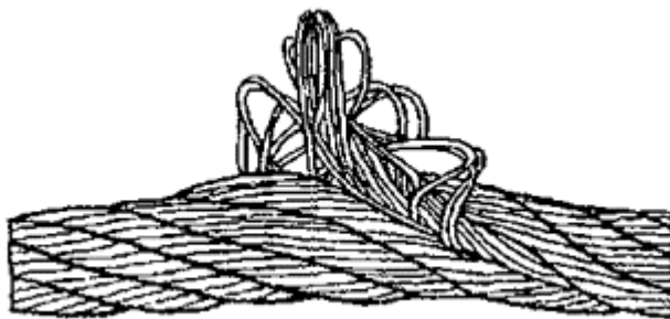
Рис. 11. Выдавливание сердечника
